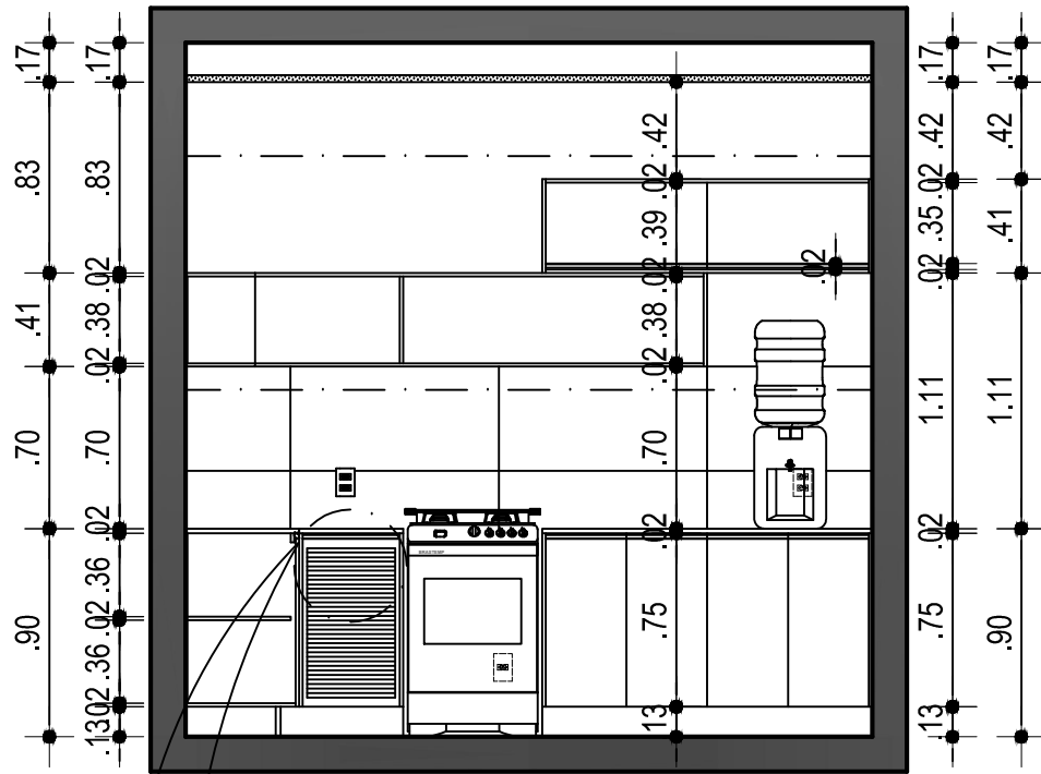
VISTA A-A' - Técnica ESCALA : ----- 1/25
