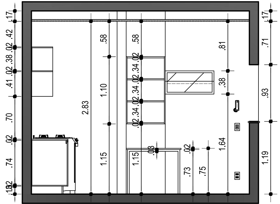
VISTA B-B' - Técnica ESCALA : ----- 1/25
