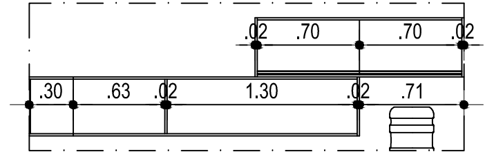
DETALHAMENTO - ARMÁRIO
