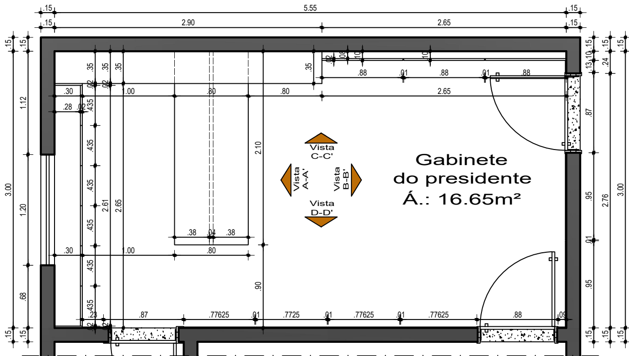
PLANTA BAIXA - Técnica ESCALA : ----- 1/25
