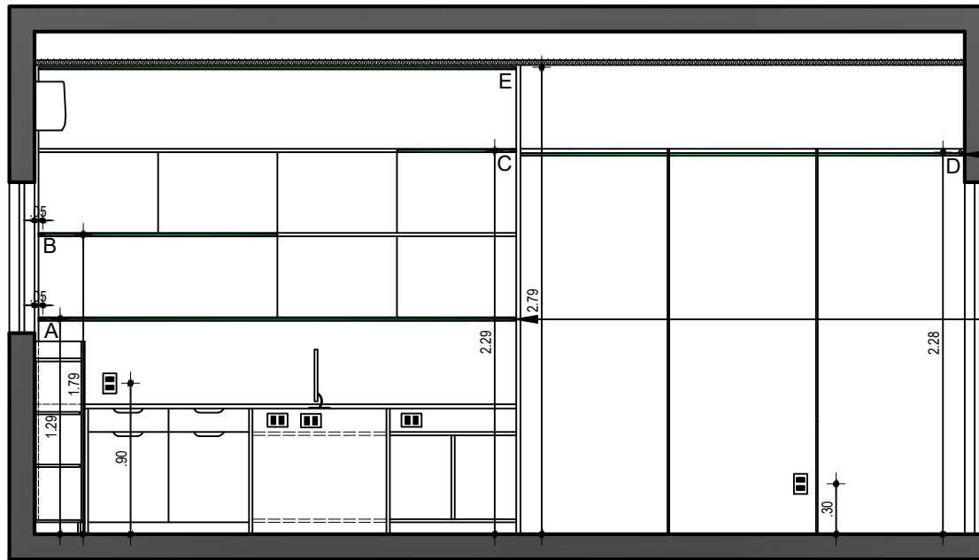
VISTA B-B' - Pontos p/ fios energizados
